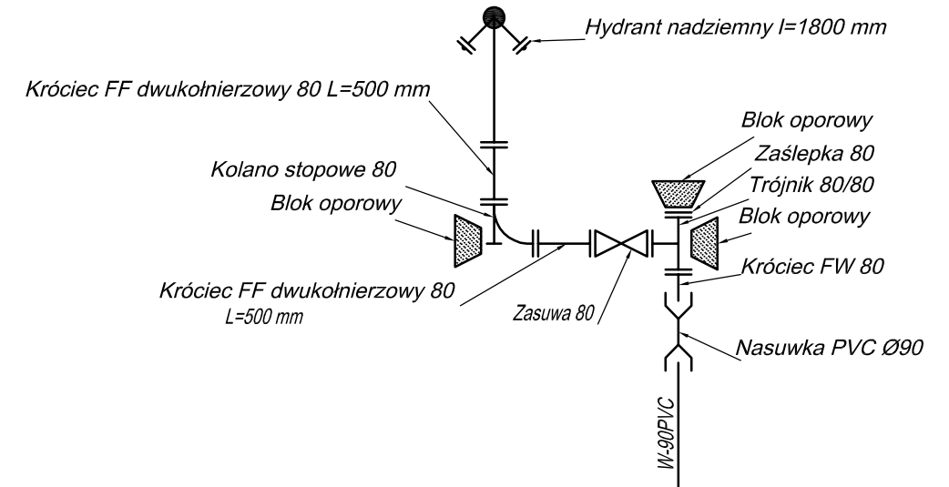
WĘZEŁ W29, HP2
