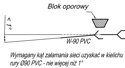
WĘZEŁ W6, W7, W8, W11, W5.2
