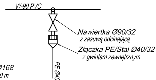
WĘZEŁ W21, W23, W24, W28
