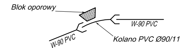
WĘZEŁ W16, W20, W25, W26
