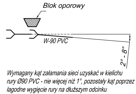
WĘZEŁ W9, W10, W12, W13, W17, W22
