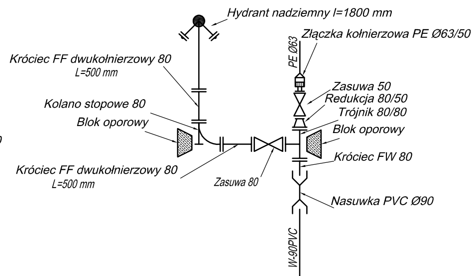
WĘZEŁ W5.4, HP1
